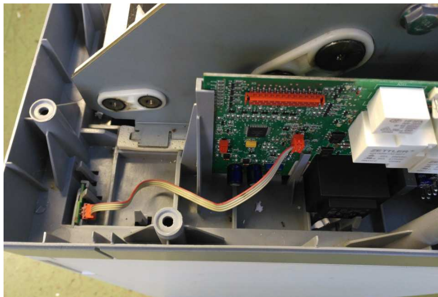
Steuerplatine in den Halter einsetzen
