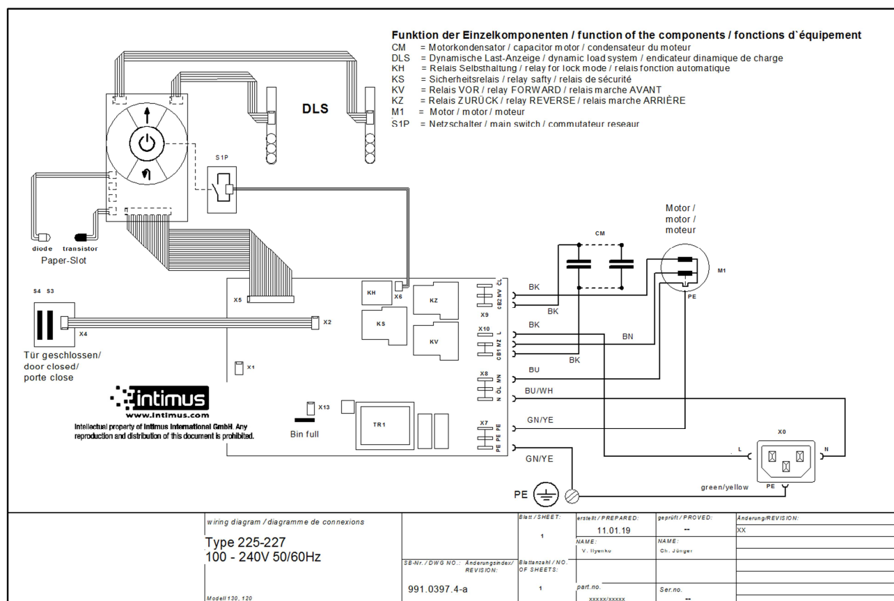
Abb. 1. Maschinenschaltbild
