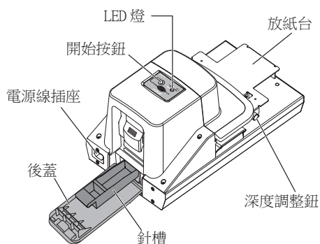
〔主機後部〕
