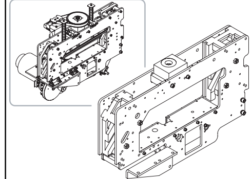
Fig.20 Frame(NewType) / 断裁フレーム(新)
