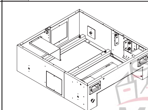
Fig.11 Chassis / シャーシ
