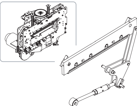
Fig.6 Knife&Drive / カッター&駆動
