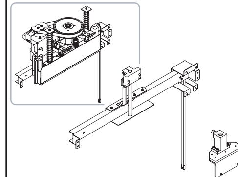
Fig.8 Clamp(2) / プレス部(2)
