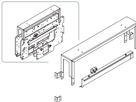
Fig.21 Cover Stay(NewType) / カバーステー(新)
