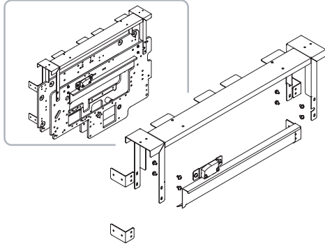
Fig.17 Cover Stay / カバーステー
