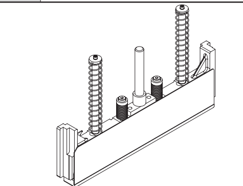
Fig.10 Clamp(4) / プレス部(4)
