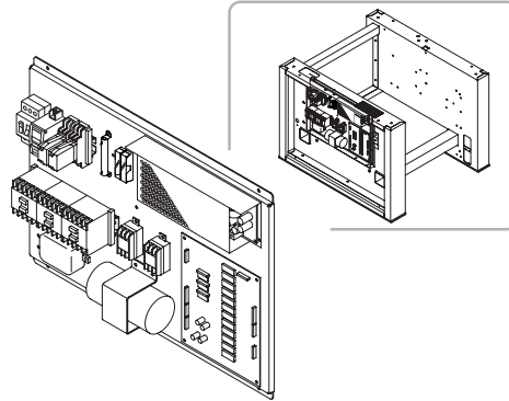
Fig.14 Electrical Parts / 電装部
