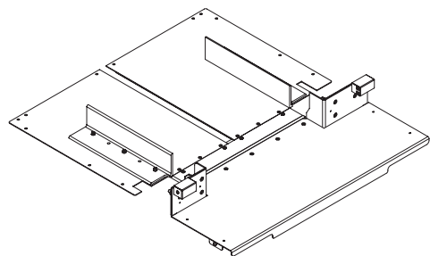
Fig.1 Table / テーブル
