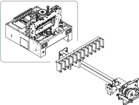
Fig.2 Backgauge / バックゲージ
