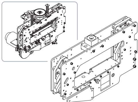
Fig.5 Frame / 断裁フレーム
