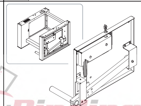
Fig.12 Foot Pedal / ペダル
