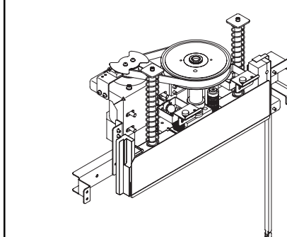
Fig.7 Clamp(1) / プレス部(1)
