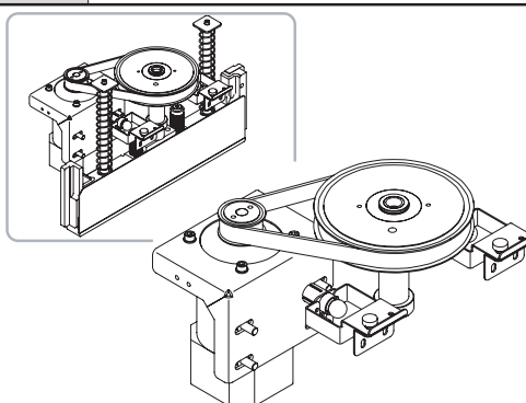
Fig.9 Clamp(3) / プレス部(3)
