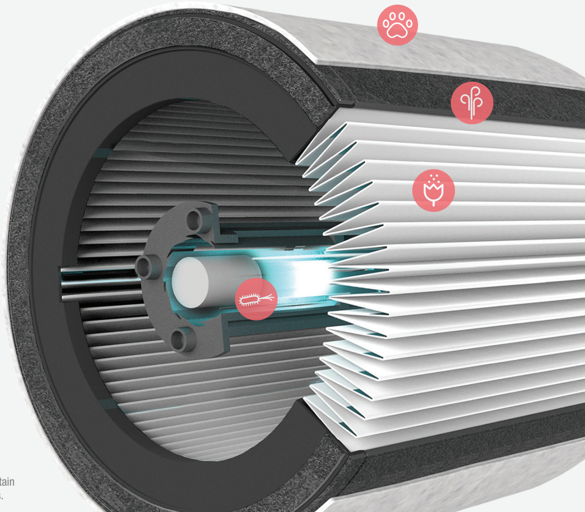
WASHABLE PREFILTER
